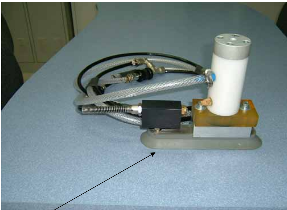
バキュームクランプシステムVTC-10 + ビストンパイプレーターVTL-155 (ウレタンプレート打撃式) 任意の場所にバキュームクランプで取り付けが可能。ビストンパイプレーターと打撃用ウレタンプレートの 組合せで振動より連続的な強力な打撃を発生を目的にしたシステム。
